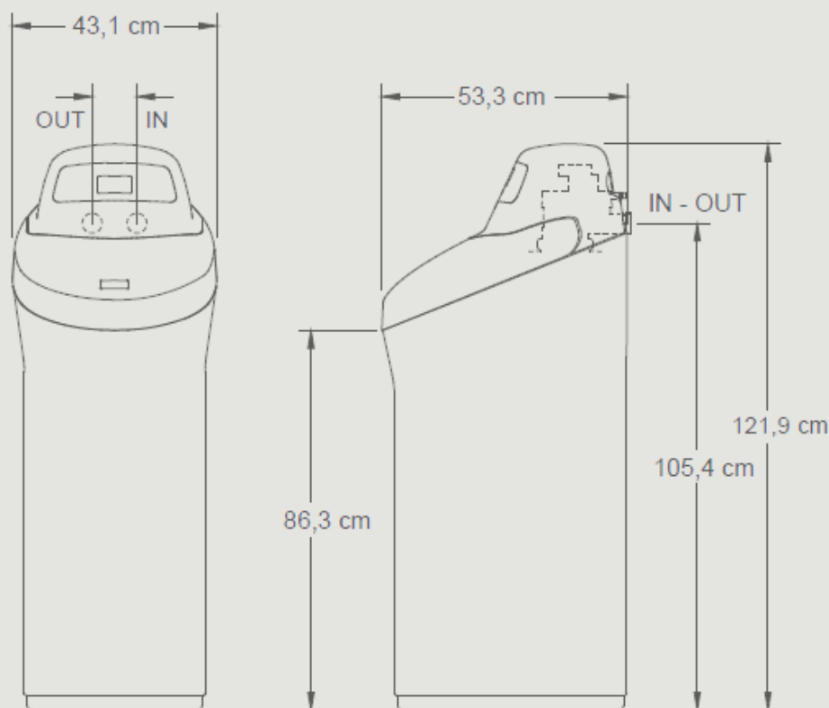
NSC42 ECOMULTI
