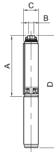
Siurblio komplekto su vienfaziu varikliu matmenys
