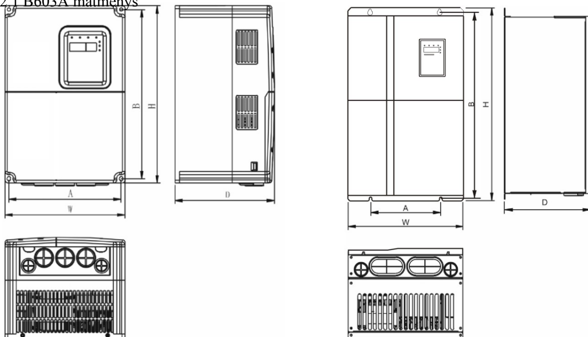
2-1-1 paveikslas. Matmenys (0,75~18,5KW) 2-1-2 paveikslas. Matmenys (22~132KW)
