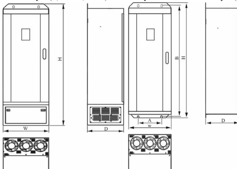
2-1-3 paveikslas. Matmenys (160~350KW)
