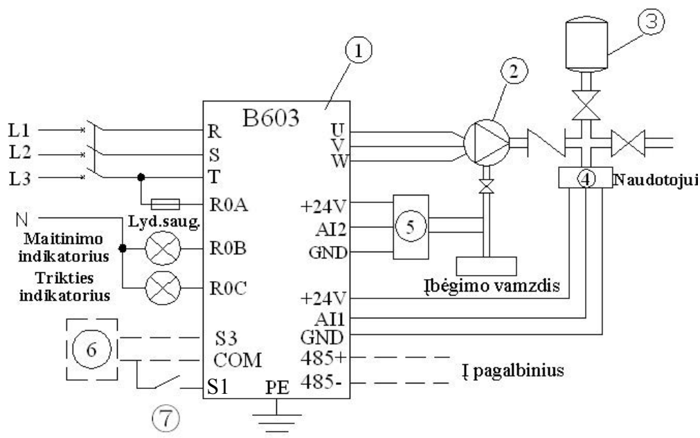
7-4-1 paveikslas. Gnybto įjungimo/išjungimo sujungimas
