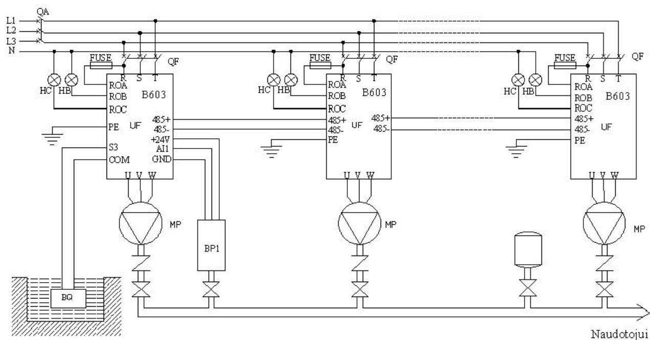
7-17-1-2 paveikslas. Kelių siurblių valdymo sujungimas
