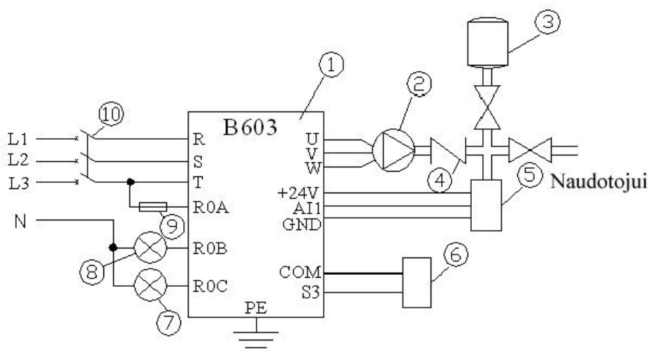
7-1-1 paveikslas. Pavienio siurblio papildomi sujungimai trikčių rodymui
