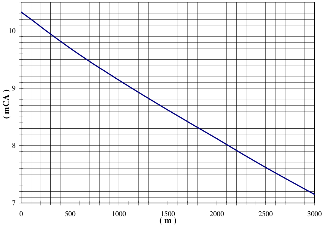
Fig. 7: pV
