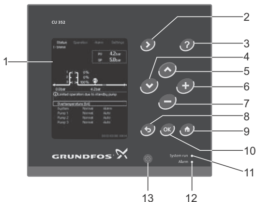
Fig. 5 CU 352 control panel
