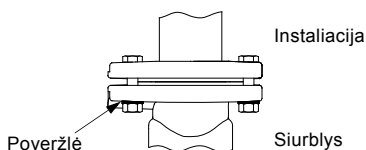
3. pav. Poveržlių naudojimas ovalinėms varžtų angoms
