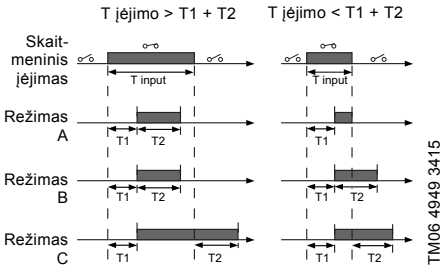
60. pav. Skaitmeninių įėjimų trukmės laikmačio veikimas
