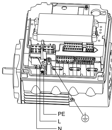
16. pav. Vienfazį variklį prijungimas prie elektros tinklo
