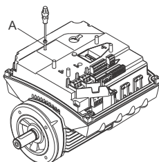
75. pav. Tvirtinimo varžto išsukimas
