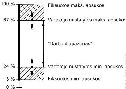
61. pav. Minimalių ir maksimalių apsukų pavyzdys
