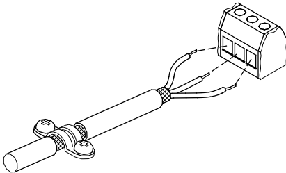
20. pav. Kabelis su prijungtu ekranu ir laidais
