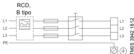
17. pav. Variklio, prijungto prie tinklo su įvadinio kirtiklio, saugikliu ir papildoma apsauga, pavyzdys
