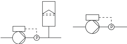
42. pav. "Pastovus slėgis"
