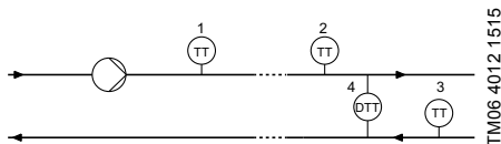
57. pav. Galimos Pt100/1000 jutiklių vietos
