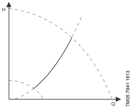
51. pav. "Pastovus lygis"
