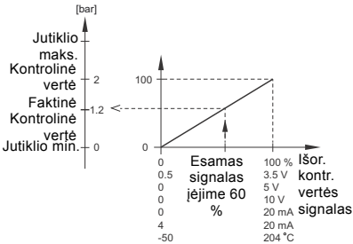
62. pav. Kontrolinės vertės korekcijos su jutiklio signalu pavyzdys
