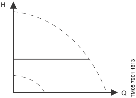
41. pav. "Pastovus slėgis"
