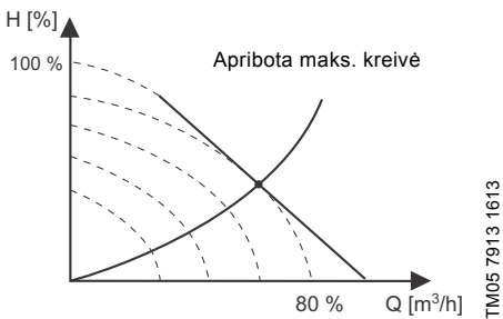
54. pav. Maks. kreivė su galios ir slėgio apribojimais
