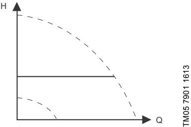
45. pav. "Pastovus diferencinis slėgis"
