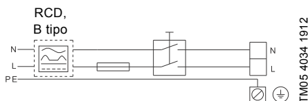
15. pav. Variklio, prijungto prie tinklo su įvadinio kirtiklio, saugikliu ir papildoma apsauga, pavyzdys
