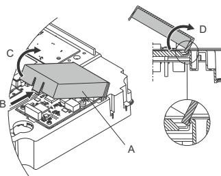
74. pav. CIM dangtelio nuėmimas
