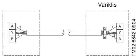
22. pav. Prijungimas ekranuotu 2 gyslų kabeliu
