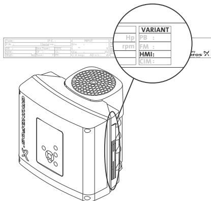
81. pav. Valdymo skydelio identifikavimas
