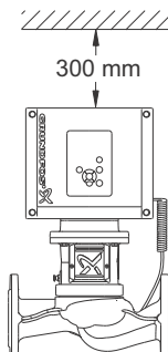
4. pav. Tarpas, kurį reikia palikti virš variklio
