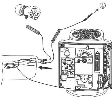
72. pav. Antistatinis remonto komplektas
