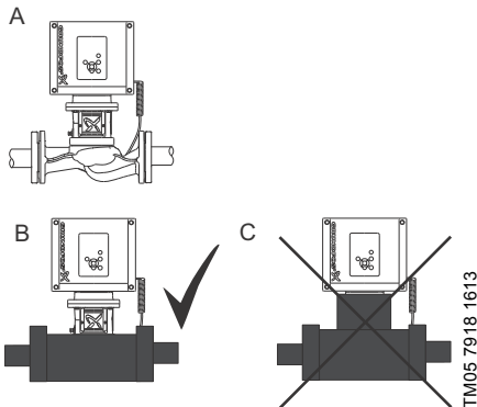
12. pav. TPE2 ir TPE3 siurbių izoliavimas
