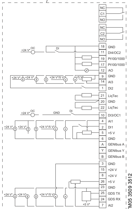
19. pav. FM 300 (pasirinktinė įranga) prijungimo gnybtai
