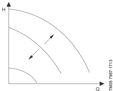
53. pav. "Pastovi kreivė"
