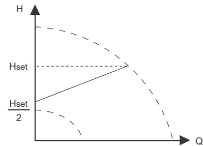
39. pav. "Proporcinis slėgis"
