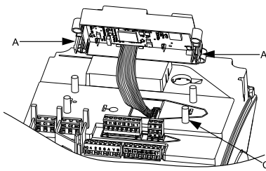
86. pav. Plastinio dangtelio uždėjimas
