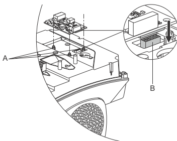
76. pav. CIM modulio įdėjimas
