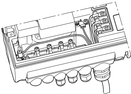
8. pav. Du apsauginio įžeminimo laidai panaudojant du 5 gyslų maitinimo kabelio laidas
