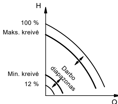
28. pav. Min. ir maks. apskukų nustatymas procentais nuo maksimalių apskukų
