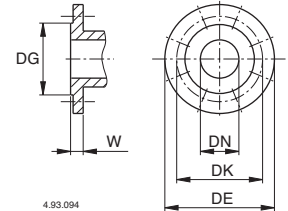
Flanges PN 10, EN 1092-2
