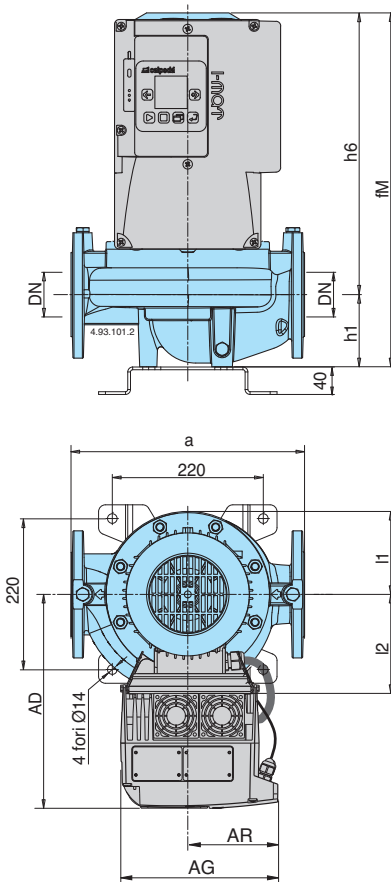
Flanges Bridas PN 10, EN 1092-2
