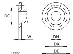
Flanges Bridas PN 10, EN 1092-2
