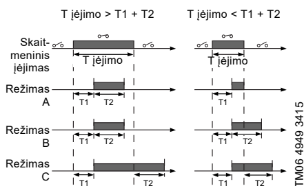
43. pav. Skaitmeninių jėjimų trukmės laikmačio veikimas
