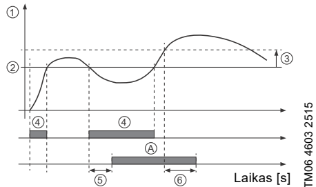
51. pav. Reagavimas į ribinės vertės viršijimą (pavyzdys)
