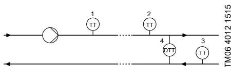
40. pav. Galimos Pt100/1000 jutiklių vietos
