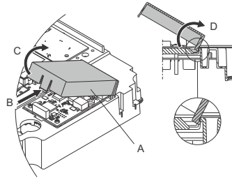
56. pav. CIM dangtelio nuėmimas
