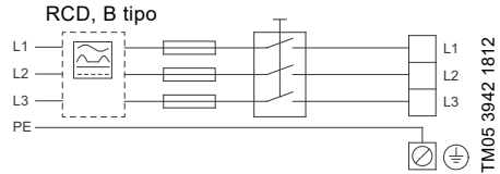
6. pav. Variklio, prijungto prie tinklo su įvadiniu kirtikliu, saugikliais ir papildoma apsauga, pavyzdys
