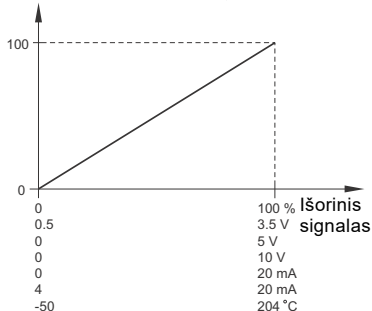
47. pav. Tiesinė funkcija
