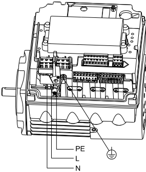
5. pav. Vienfazių variklių prijungimas prie elektros tinklo
