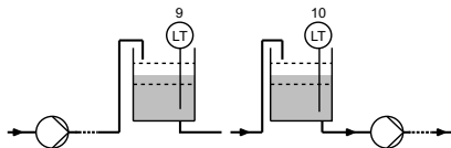
39. pav. Galimos jutiklių vietos
