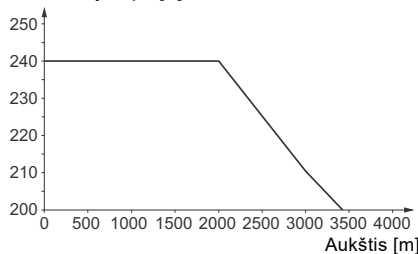
14. pav. Vienfazių variklių maitinimo įtamos priklausomybė nuo aukščio virš jūros lygio
