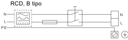
4. pav. Variklio, prijungto prie tinklo su įvadiniu kirtikliu, saugikliu ir papildoma apsauga, pavyzdys
