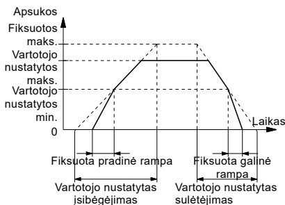
52. pav. Įsibėgėjimas ir sustojimas
