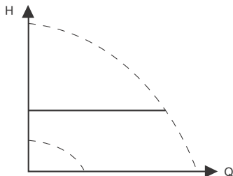
30. pav. "Pastovus diferencinis slėgis"
