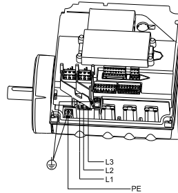
7. pav. Trifazių variklių prijungimas prie elektros tinklo
