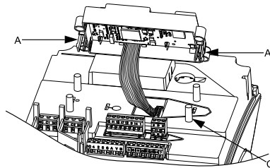
68. pav. Plastikinio dangtelio uždėjimas
