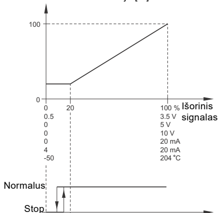
48. pav. Tiesinė su stop
