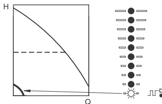
19. pav. Min. kreivės režimas
