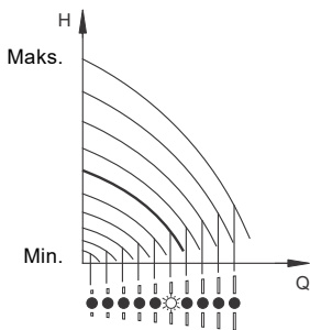
17. pav. Siurblys pastovios kreivės valdymo režime
