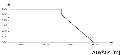
13. pav. Trifazių variklių maitinimo įtamos priklausomybė nuo aukščio virš jūros lygio
