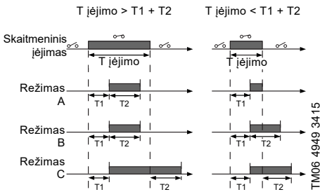
41. pav. Skaitmeninių įėjimų trukmės laikmačio veikimas
