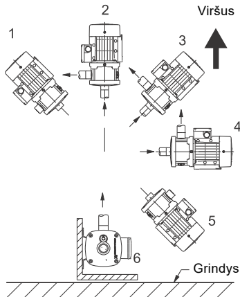
1. pav. Siurblio padėtytys
