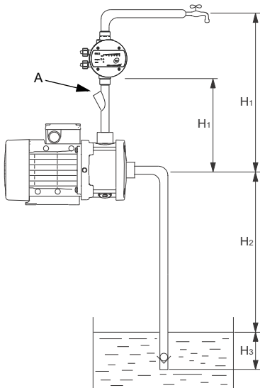
4. pav. Savisiurbiui siurbliui rekomenduojami vamzdžiai
