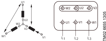
11 pav. Prijungimas žvaigžde
