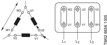
10 pav. Prijungimas trikampiu
