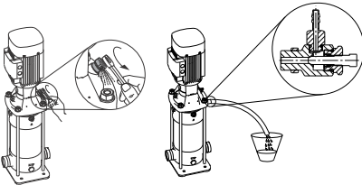
16 pav. Oro išleidimo vožtuvas, standartinis ir pasirenkamas sprendimas su jungtimi žarnai
