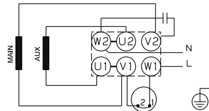
15 pav. 240 V, 1,1 - 2,2 kW prijungimas
