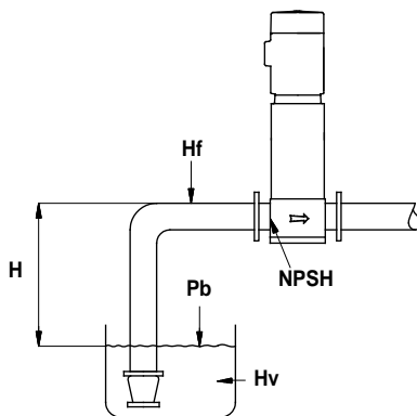
21 pav. Principinė atviros sistemos su CR siurbliu schema
