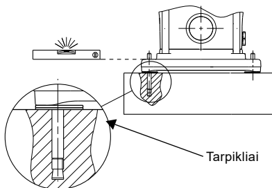
6 pav. Išlyginimas tarpkliais
