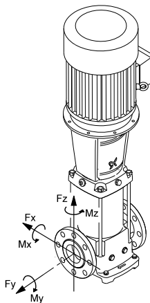
9 pav. Flanšus veikiančios jėgos ir jėgos momentai
