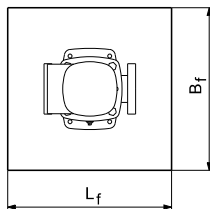
3 pav. Pamatą, vertikalus montavimas
