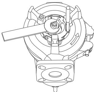
14. pav. Darbaračio tarpelio reguliavimas
