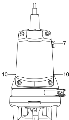
13. pav. Lygio ir sausosios eigos jutiklių vieta
