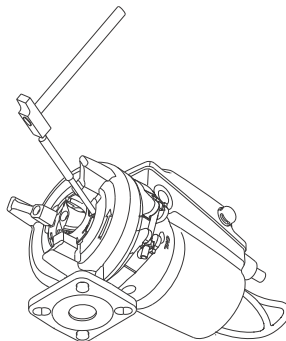
15. pav. Smulkinimo žiedo nuėmimas
