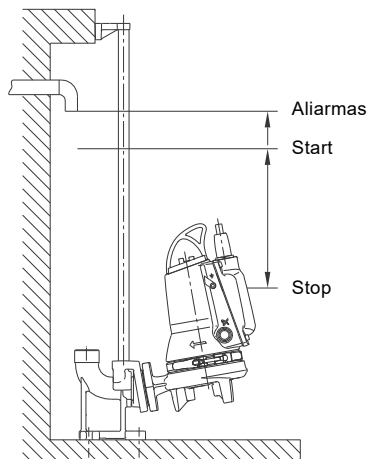
6. pav. Paleidimo ir stabdymo lygiai
