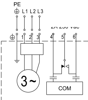
3. pav. Trifazių siurblių prijungimo schema
