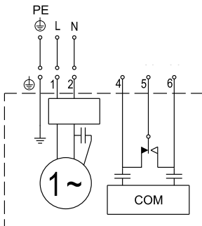
2. pav. Vienfazių siurblių prijungimo schema
