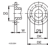
Flanges PN 10, EN 1092-2
