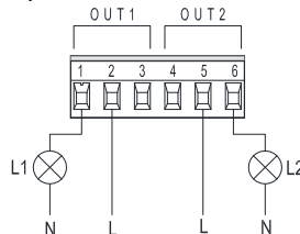
Εικόνα 9: Αφαιρούμενη κλέμμα 6 πόλων: παράδειγμα σύνδεσης εξόδων
