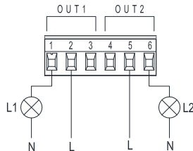
Схема 9: Изходи на 6-пинов терминал: примерна изходяща връзка
