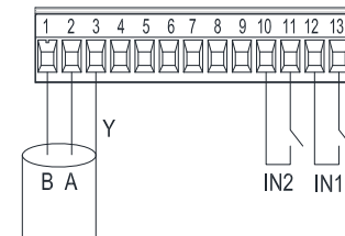
Figura 7: Terminal de bornes extraíble 13 polos: entradas digitales y MODBUS
