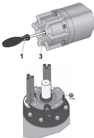
Figure 5-5 : Contrôle du liquide moteur
