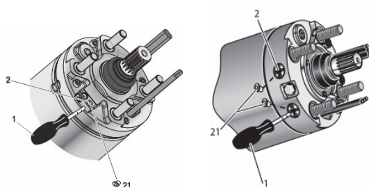
Figura 5-2: motore da 6", 8", 10"
