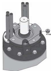
Ilustración 5-5: Control del líquido del motor
