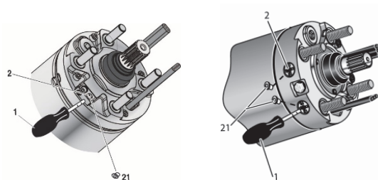
Εικόνα 5-2: κινητήρας 6", 8", 10"
