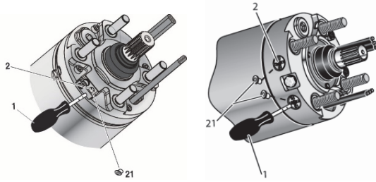
Resim 5-2: Motor 6'', 8'', 10''
