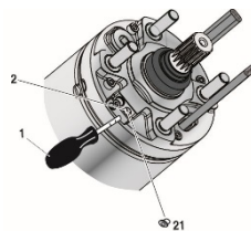
Bild 5-2: Motor 6", 8", 10"
