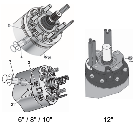
Figura 5-6: rabboccatura del liquido del motore
