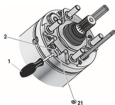
Ilustración 5-2: Motor de 6", 8", 10"
