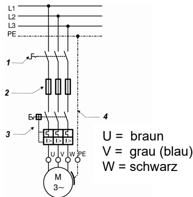
Bild 5-10: Absicherung und Motorschutz
