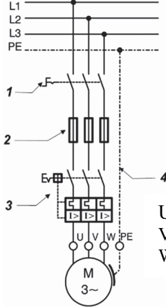
Resim 5-10: Sigorta ve motor koruyucu
