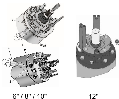
Bild 5-5: Motorflüssigkeit kontrollieren
