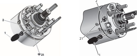
Figure 5-2 : Moteur 6" / 8" / 10"
