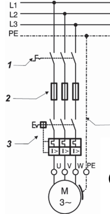
شكل 5 - 10: تركيب المصاهر وحماية المحرك
