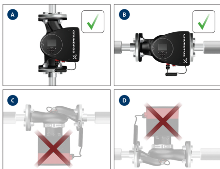
Siurblys turi būti sumontuotas taip, kad variklio velenas būtų horizontalus
