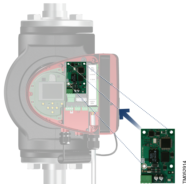
CIM modulio vieta MAGNA3 siurblyje
