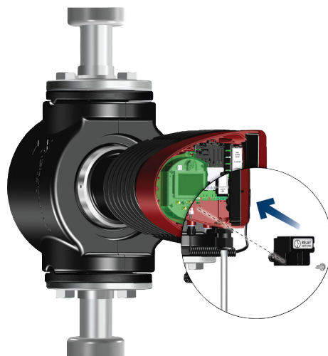
Relių dangtelio ir varžto uždėjimas
