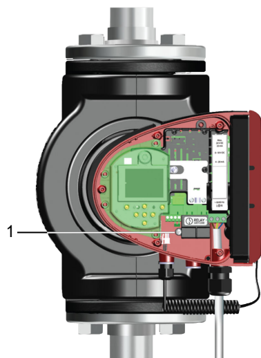
Relių dangtelio (1 poz.) atsukimas
