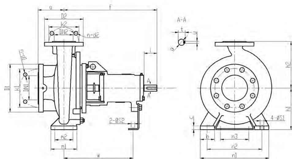
DN1/DN2 32 40 50 65 80 100 125 150 200 250 300 350 400 D1/D2 140 150 165 185 200 220 250 285 340 405 460 520 580 K1/K2 100 110 125 145 160 180 210 240 295 355 410 470 525 n-d1/n-d2 4-Φ18 4-Φ18 4-Φ18 4-Φ18 8-Φ18 8-Φ18 8-Φ18 8-Φ22 12-Φ22 12-Φ26 12-Φ26 16-Φ26 16-Φ30
