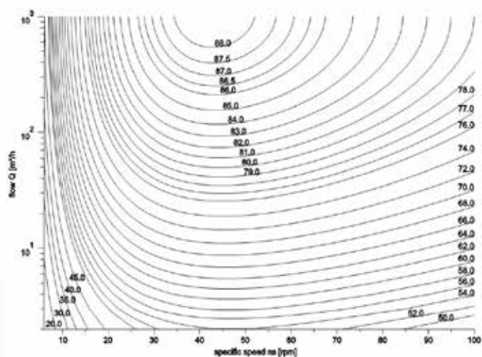
MEI = 0.7 for ESOB 1450 rpm
